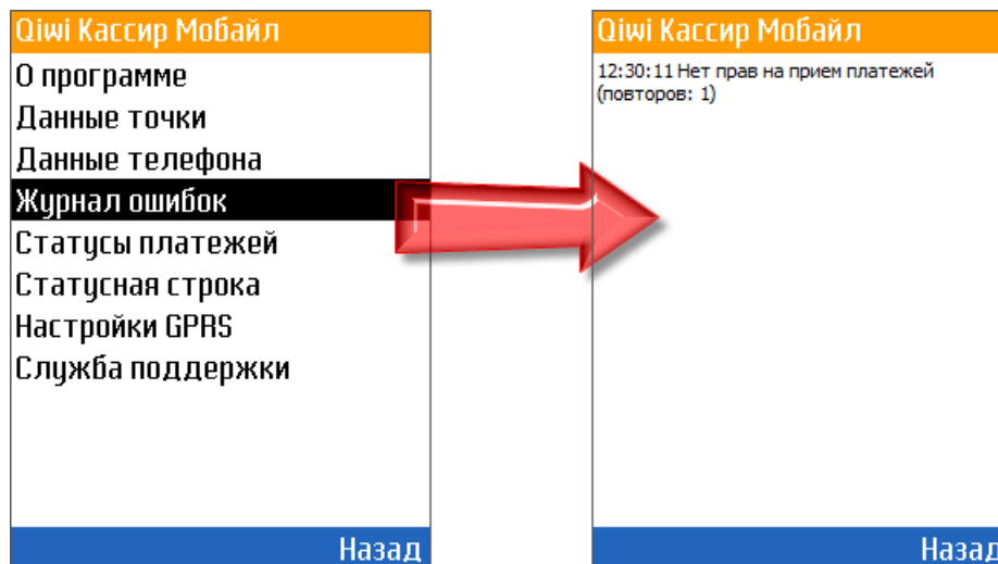
Рис. 22. Журнал ошибок
